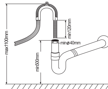
Anschließen des Wasserauslassschlauchs
