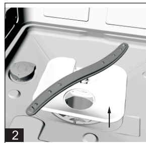
Schritt 2: Heben Sie den Flachfilter an
