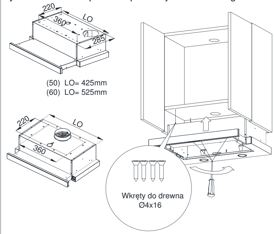
Rys. 5d Montaż korpusu okapu wersja mocowanie górne.
