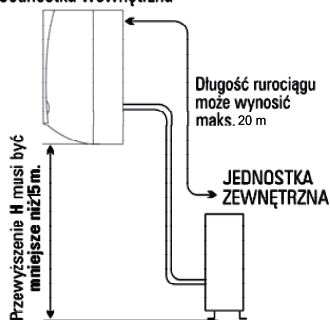
Jednostka wewnętrzna
