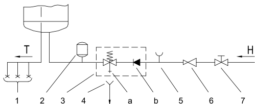
Слика 2: Затворен систем (со притисок)
