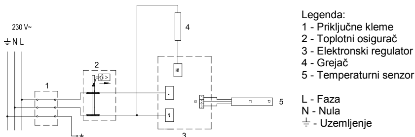
Sl. 5: Šema povezivanja električnih provodnika
