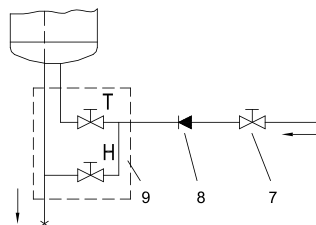
Слика 3: Отворен систем (прелевен)
