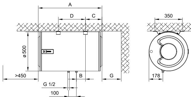
Sl. 1: Horizontalna namestitev na strop
