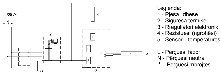
Fig. 5: Skema e lidhjes elektrike
