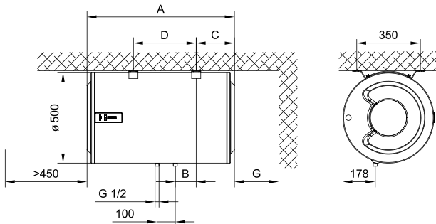
Abb. 1: Horizontale Installation an der Decke
