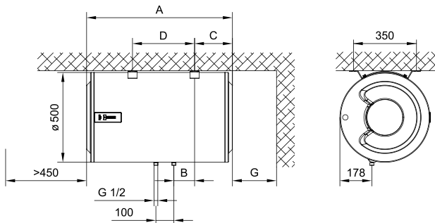
Fig. 1: Instalimi horizontal në tavan
