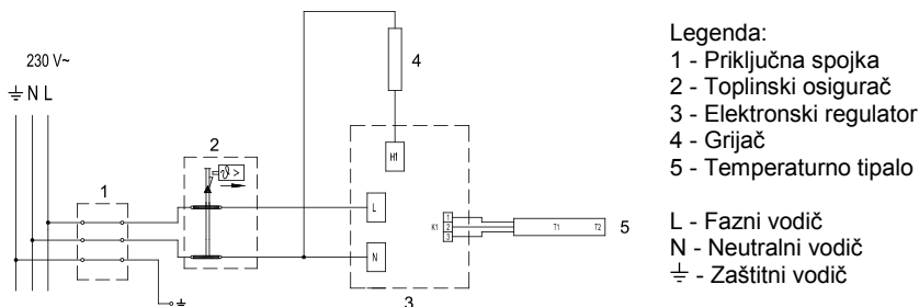
Sl. 5: Električna spojna shema
