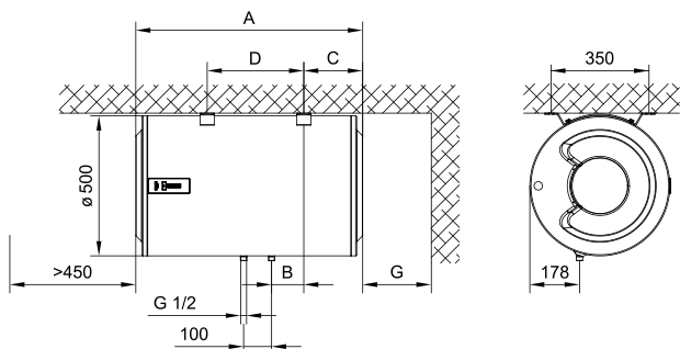
Sl. 1: Vodoravno postavljanje na strop
