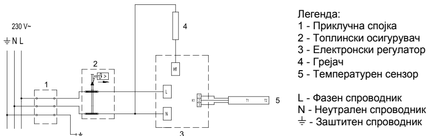
Сл. 5: Шема на електрично поврзување
