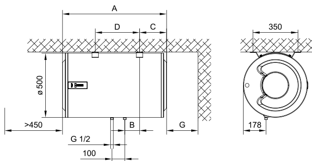
Сл. 1: Хоризонтално местење на плафон
