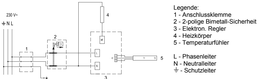
Abb. 5: Elektroschaltbild
