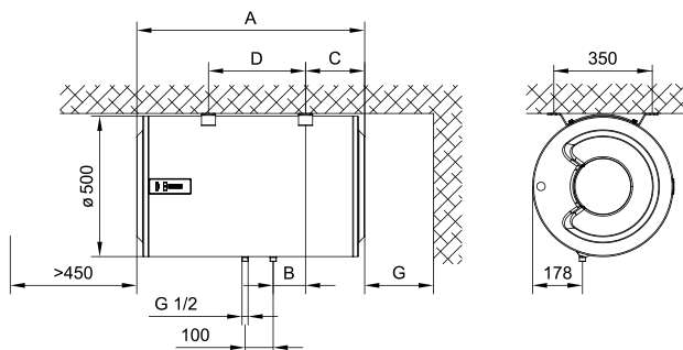
Sl. 1: Vodoravna montaža na plafon
