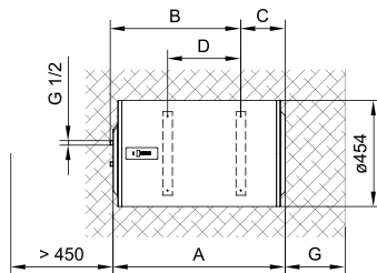
Sl. 2: Vodoravna namestitvev na steno
