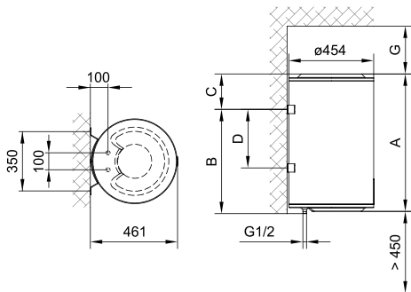
Fig. 1: Montimi vertikal në mur
