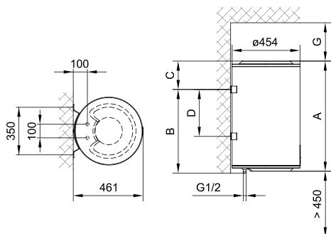
Sl. 1: Pokončna namestitvev na steno
