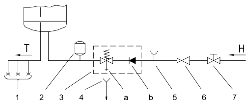
Fig. 3: Sistemi i mbyllur (me presion)
