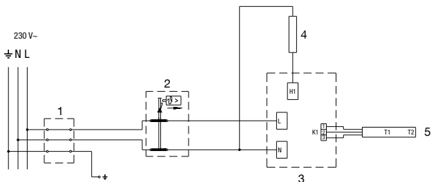
SI. 5: Električna spojna shema
