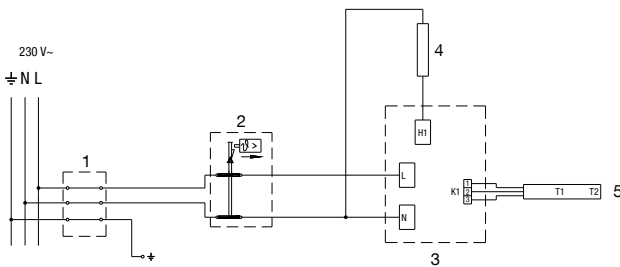
Fig. 5: Skema e lidhjes elektrike
