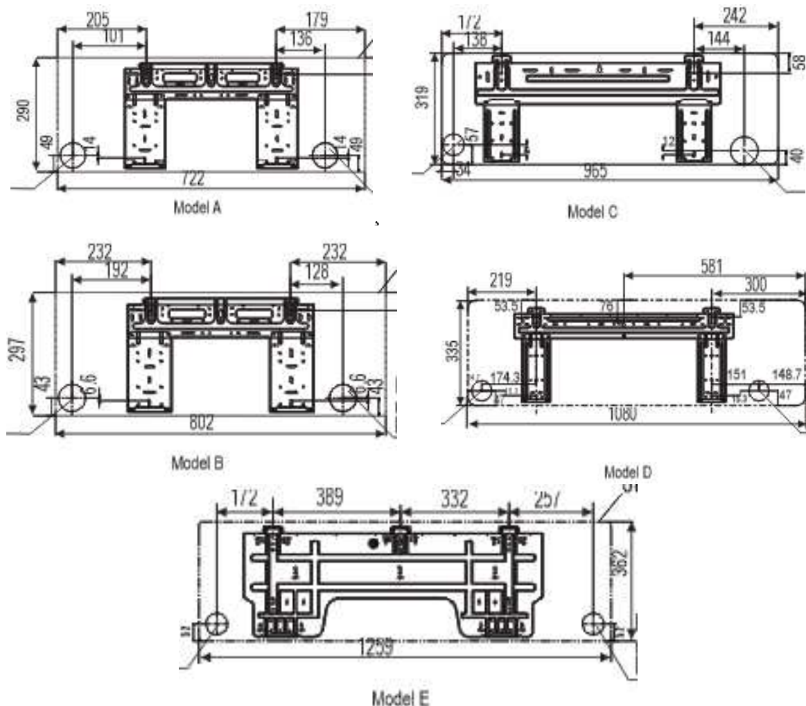
Slika 5: Priporočene pozicije lukenj za plinsko in električno povezavo KAS26SDCINVA, KAS35SDCINVA, KAS53SDCINVA
