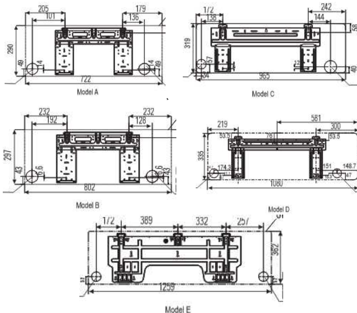
Slika 5. Preporučljivi položaji rupa za plinsko i električno povezivanje KAS26SDCINVA, KAS35SDCINVA, KAS53SDCINVA
