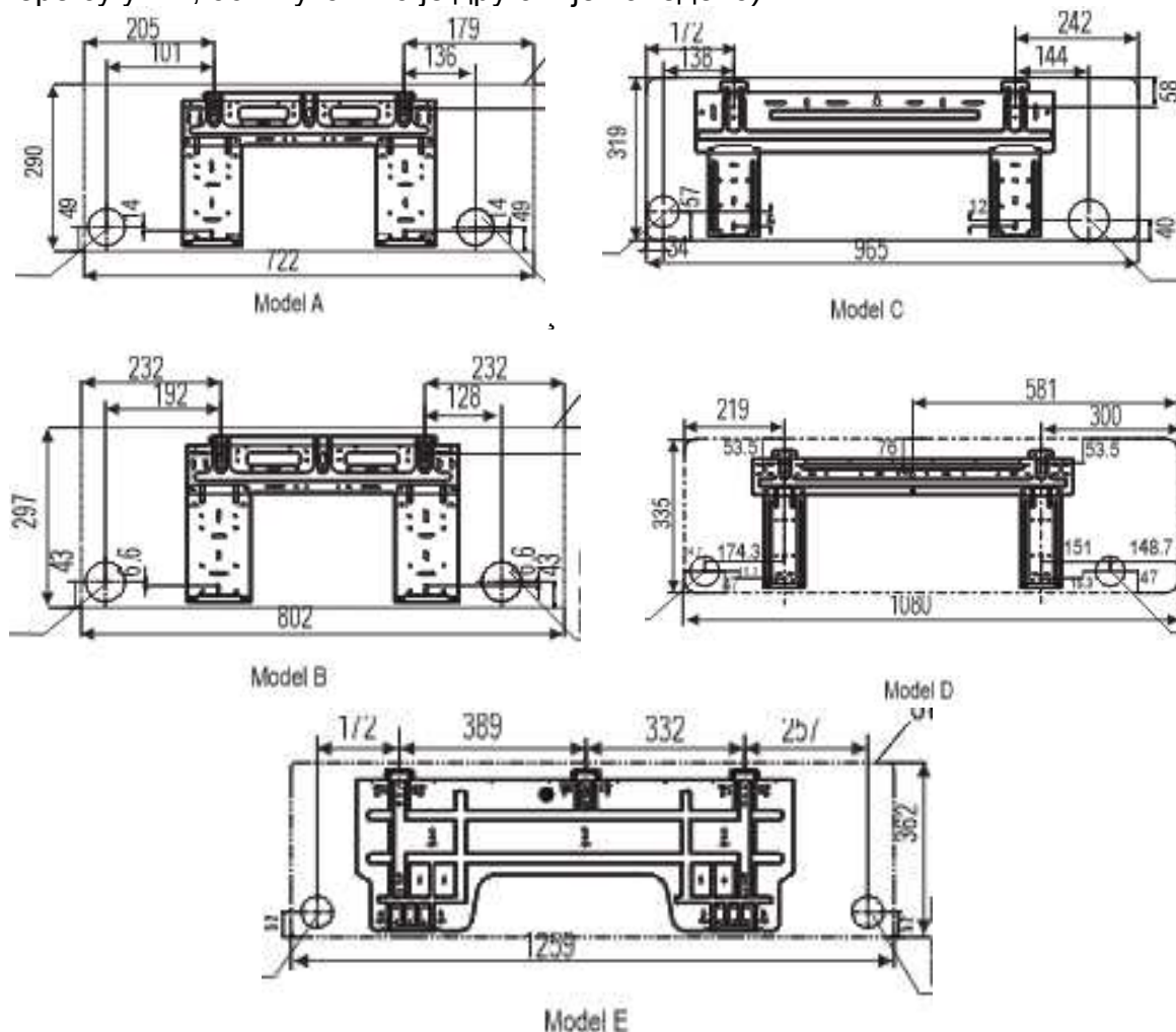
Слика 5. Препоручљиви положаји рупа за гасно и електрично повезивање KAS26SDCINVA, KAS35SDCINVA, KAS53SDCINVA
