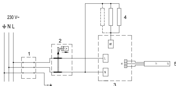
Sl. 5: Shema električne vezave
