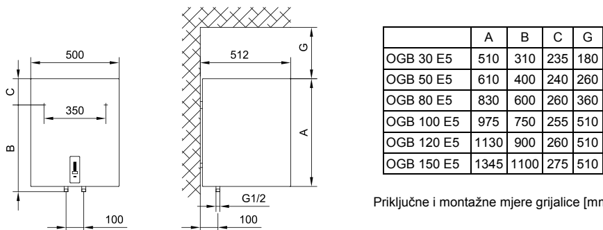
Sl. 1: Uspravno postavljanje na zid
