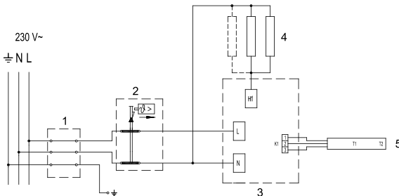
Abb. 5: Elektroschaltbild
