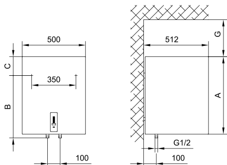
Sl. 1: Pokončna namestitvev na steno
