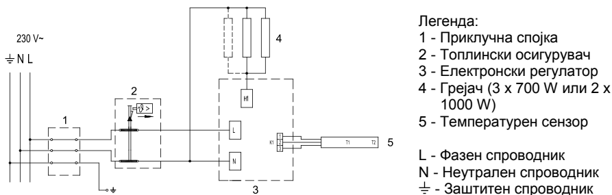
Слика 5: Шема на електрично поврзување
