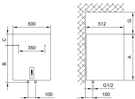
Сл. 1: Исправено поставување на сид
