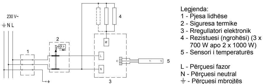
Fig. 5: Skema e lidhjes elektrike
