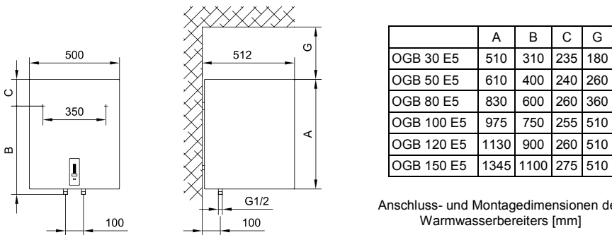
Abb. 1: Senkrechte Montage an die Wand
