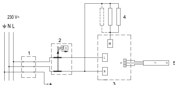
Sl. 5: Električna spojna shema
