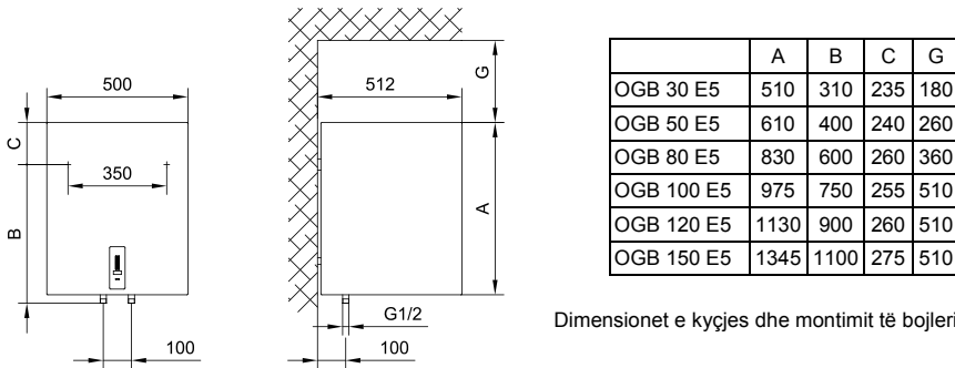
Fig. 1: Montimi vertikal në mur
