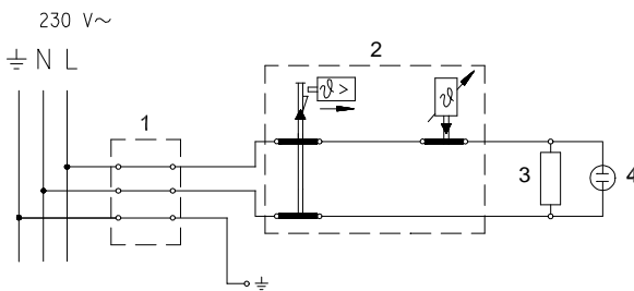
Електросхема
