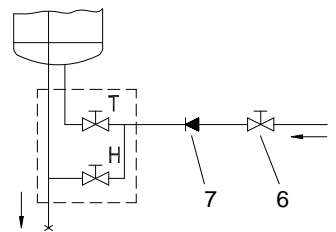
Otvoreni sistem (protočni)
