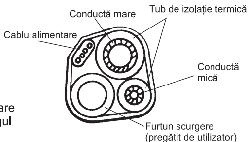
Învelire cu bandă de vinil
