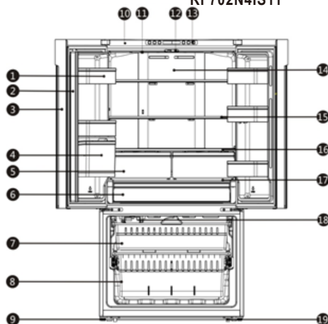
Vue 2 de l'appareil RF702N41S1 FMN544I20S RF702N41S11
