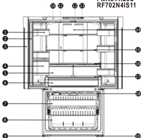
Descrizione 2 dell'apparecchio RF702N41S1 FMN544I20S RF702N41S11
