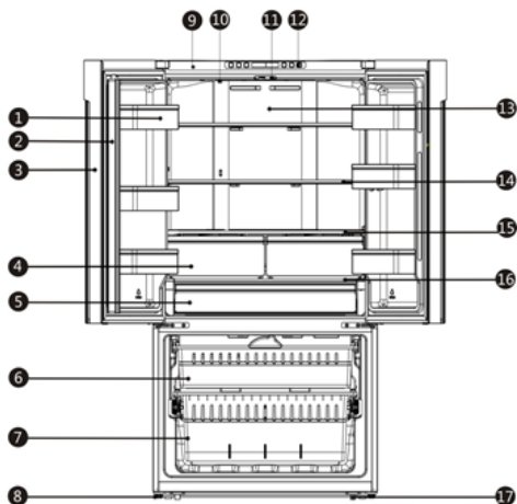
Vue 2 de l'appareil RF715N4AS1
