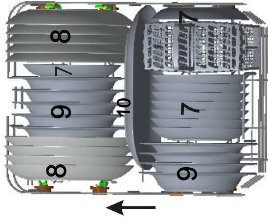
2.Coșul inferior
