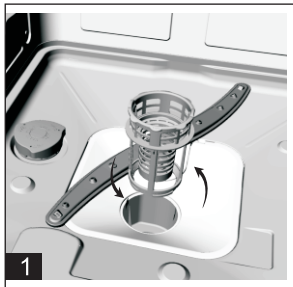
Schritt 1: Den Grobfilter kontrarotieren und dann anheben.
