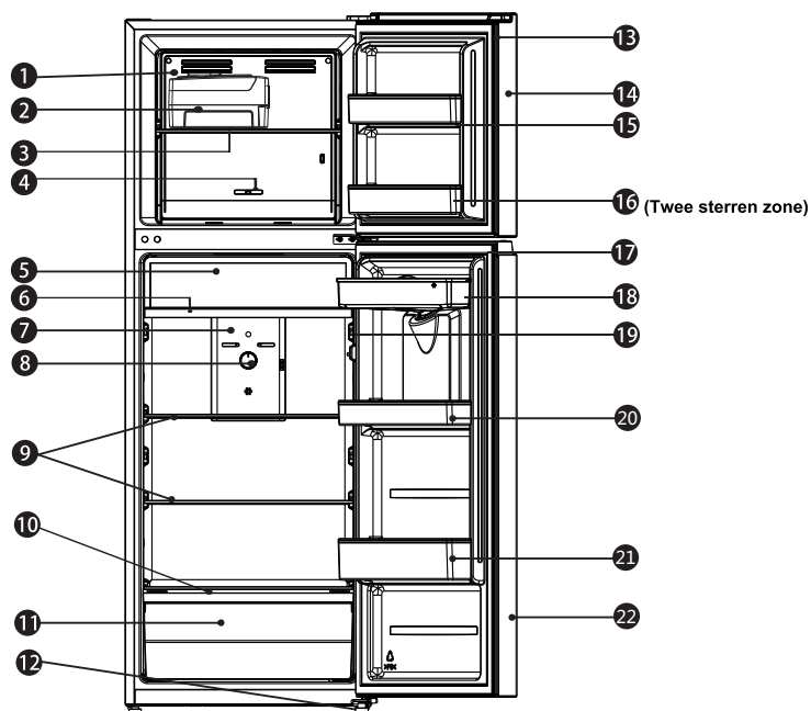
Dwarsdoorsnede van het apparaat
