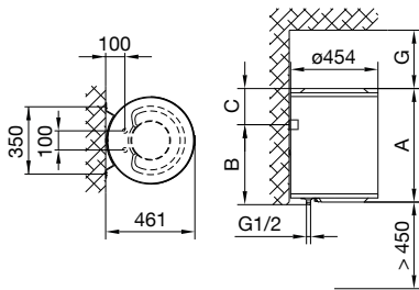
1 pav.: vertikalus tvirtinimas prie sienos
