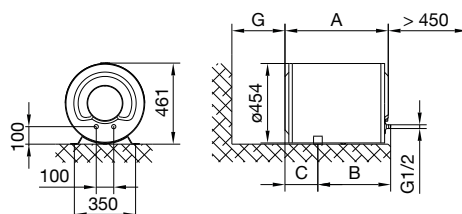
2. ábra: Vízszintes rögzítés a földre
