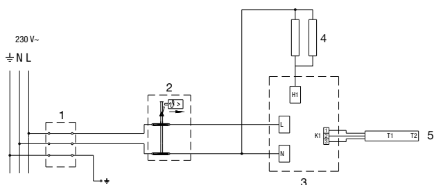
Rys. 6: Schemat podłączenia do sieci
