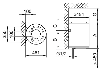
Obr. 1: Svislá instalace na stěnu
