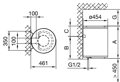
Rys. 1: Pionowy montaż na ścianie
