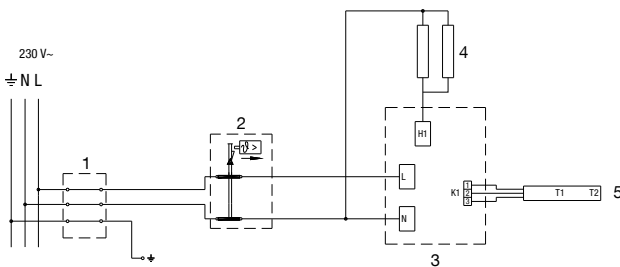
6 pav.: Elektros jungimo schema
