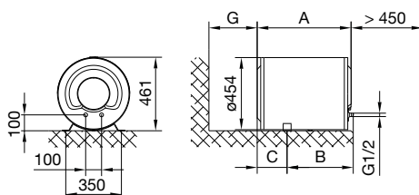
Obr. 2: Horizontální umístění na podlahu
