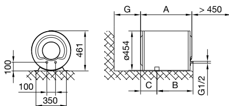
Rys. 2: Leżące umieszczenie na podłodze.
