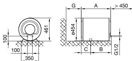
Obr. 2: Inštalácia ležmo na podlahu
