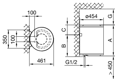
Рис. 1: Монтаж на стену в вертикальном положении
