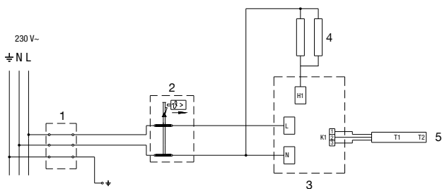
Fig. 6: Instalația electrică
