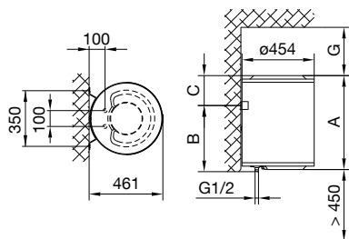
Фиг. 1: Вертикален стенен монтаж
