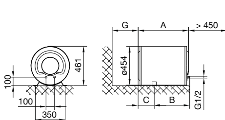
Fig. 2: Montarea orizontală pe podea
