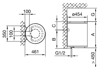
1. ábra: Függőleges felszerelés a falra
