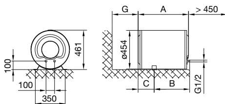
Фиг. 2: Монтаж в легнало положение на пода
