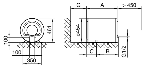
2 pav.: horizontali padėtis ant grindų
