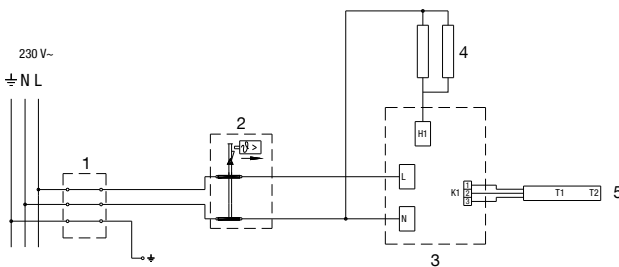
6. ábra: Elektromos bekötés vázlat
