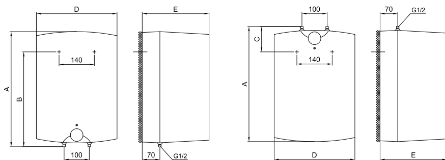
Provedení nadumyvadlové
