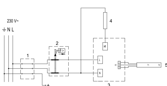
5 pav.: Elektros jungimo schema
