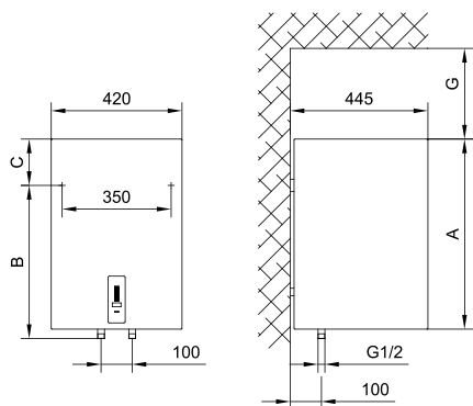
Obr. 1: Zvislá montáž na stenu
