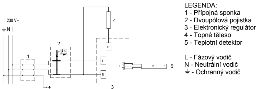
Obr. 5: Schéma elektrického připojení
