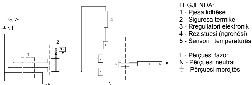
Fig. 5: Skema e lidhjes elektrike
