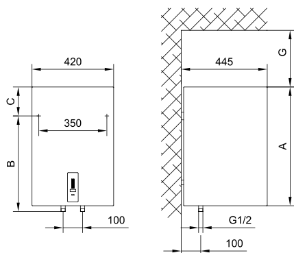
Фиг. 1: Вертикален стенов монтаж
