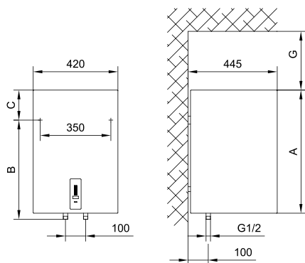
Obr. 1: Svislá instalace na stěnu
