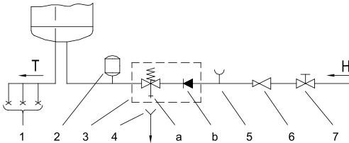
2. ábra: Zárt (nyomás alatti) rendszer
