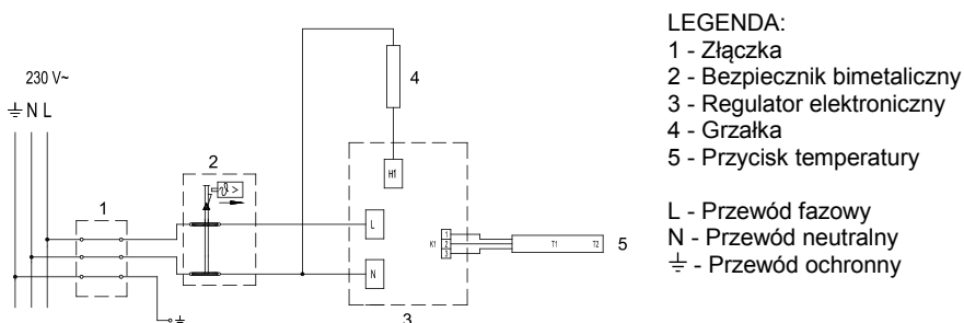
Rys. 5: Schemat podłączenia do sieci
