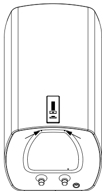
Fig. 4: Largimi i kapakut mbrojtës
