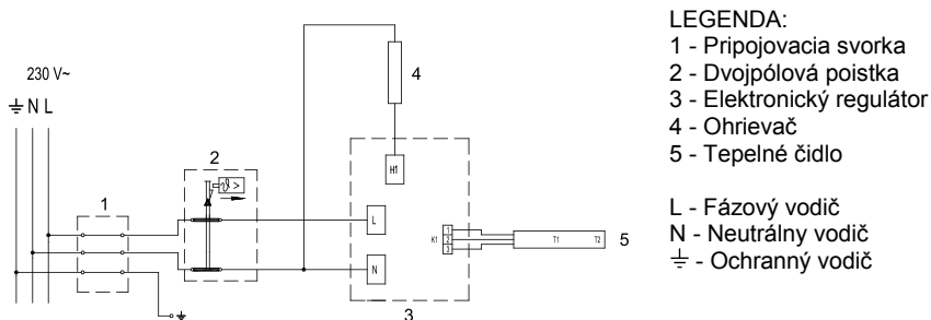
Obr. 5: Schéma elektrického pripojenia
