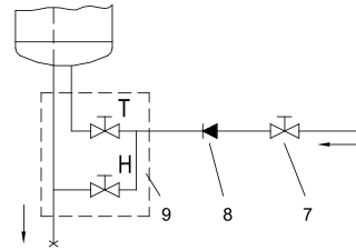
3. ábra: Nyílt (nyomás nélküli) rendszer
