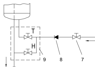
Rys. 3: Otwarty (nie ciśnieniowy) system
