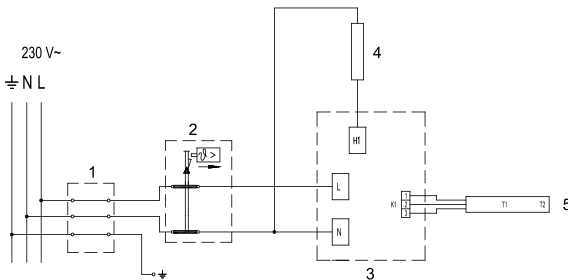
5. ábra: Elektromos bekötés vázlata
