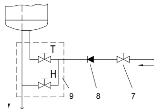
Obr. 3: Otevřený (netlakový) systém
