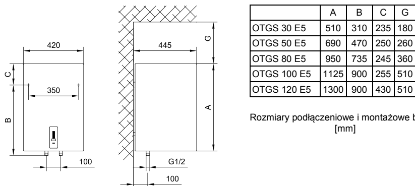
Rys. 1: Pionowy montaż na ścianie
