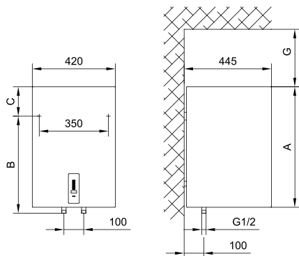
1 pav.: vertikalus tvirtinimas prie sienos
