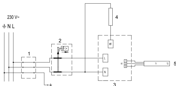
Рис. 5: Электросхема
