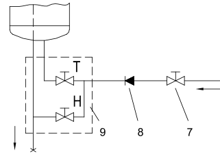
3 pav.: Atvira (pratekamoji) sistema
