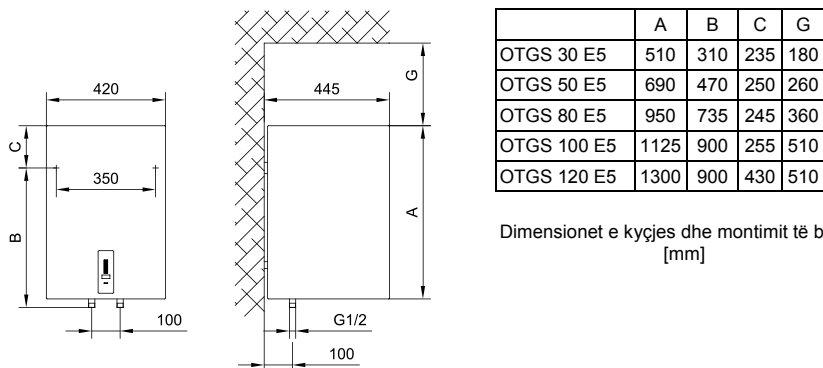
Fig. 1: Montimi vertikal në mur
