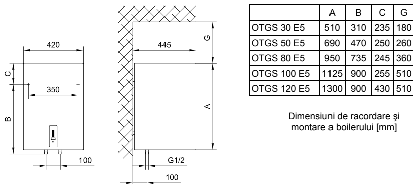
Fig. 1: Instalarea boilerului pe perete în poziție verticală
