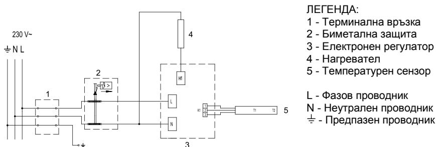
Фиг. 5: Електрическа схема
