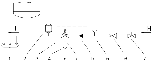
2 pav.: Uždara (kaupiamoji) sistema
