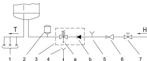
Rys. 2: Zamknięty (ciśnieniowy) system
