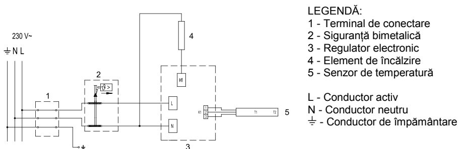
Fig. 5: Instalația electrică
