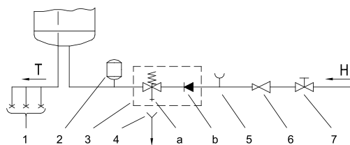
Фиг. 2: Затворена система (под налягане)
