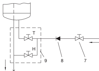
Sl. 3: Odprti (netlačni) sistem
