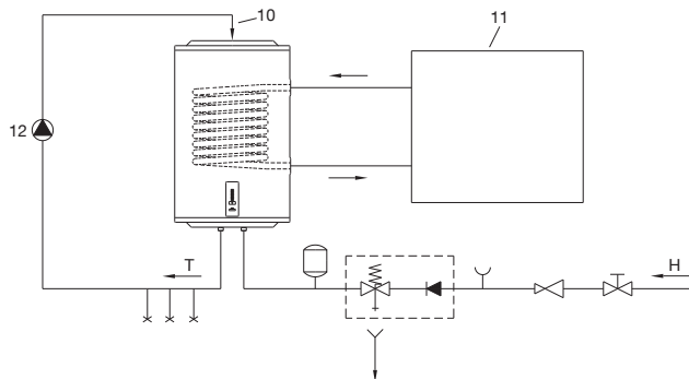
Sl. 4: Priklop grelnika na dodatni energetski vir
