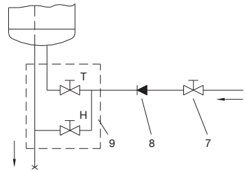
Сл. 3: Отворен систем (прелевен)
