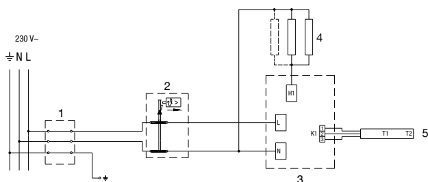
SI. 6: Električna spojna shema
