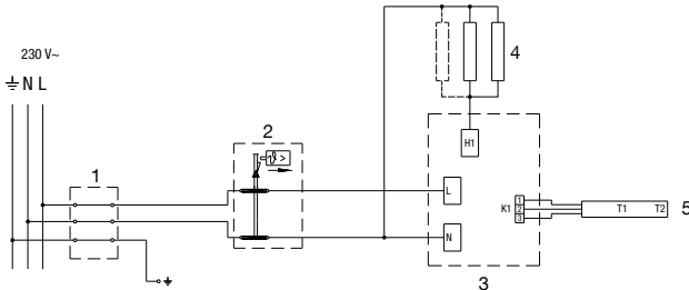
Bild 6: Elektroschaltbild
