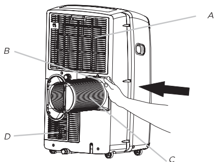
A párologtató levegő bemenet B csatlakozó elem C flexibilis kivezető cső D kondenzátor levegő bevezetés
