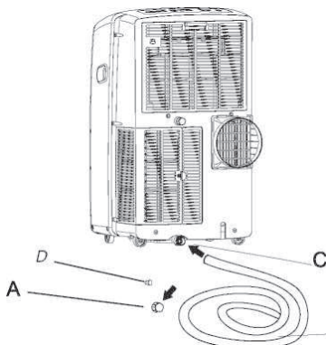
A. Port principal de scurgere B. Furtun de scurgere C. Orificiu principal de scurgere D. Dop principal de scurgere
