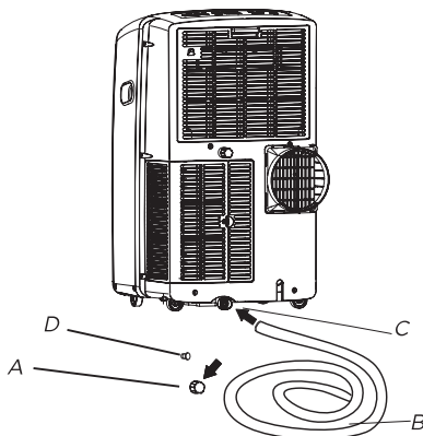
A Elsődleges vízlevezető nyílás B Vízlevezető cső C Elsődleges vízlevezető nyílás D Elsődleges vízlevezető dugasz
